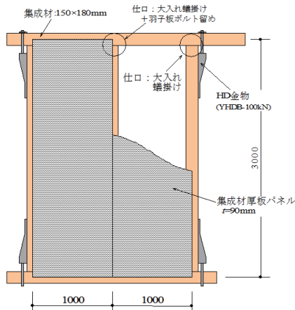
パネル間接合部の接合方法
