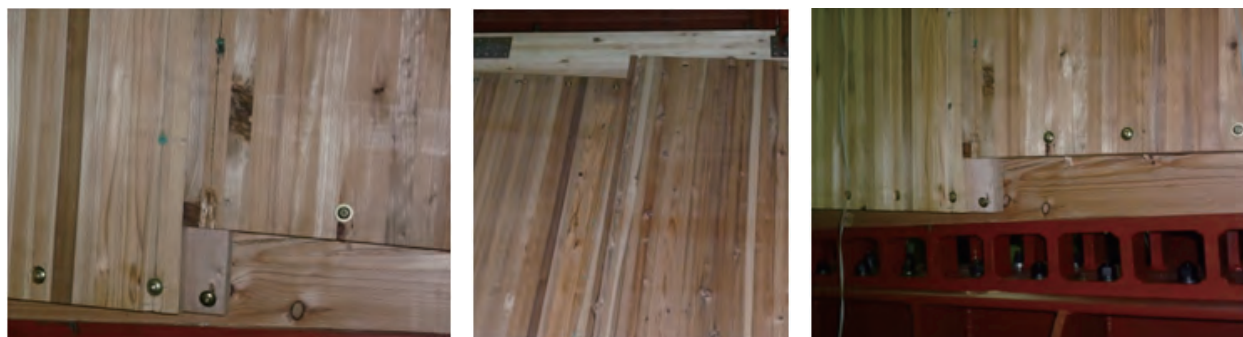
パネル間接合に変形が集中し、ビス列に沿って厚板パネルが割裂
