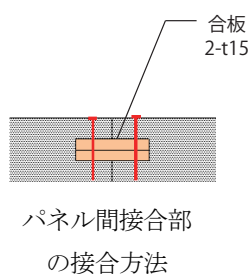
床構面試験体
