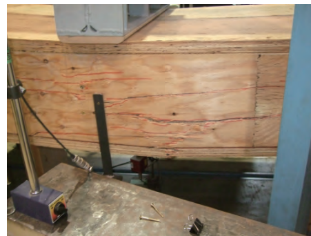
ウェブの曲げ破壊（試験体 3）
